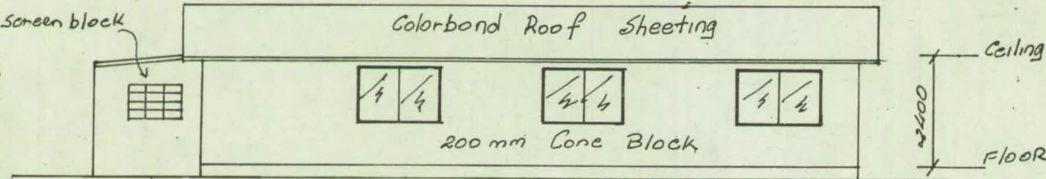
Elevation
